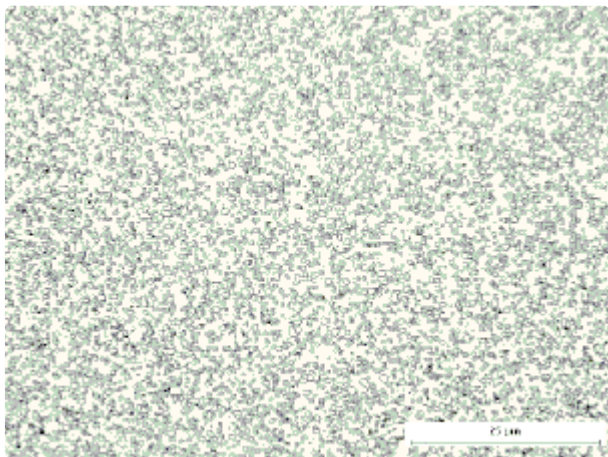
Figure 1. Alleima® 13C26 'as delivered', unhardened.
